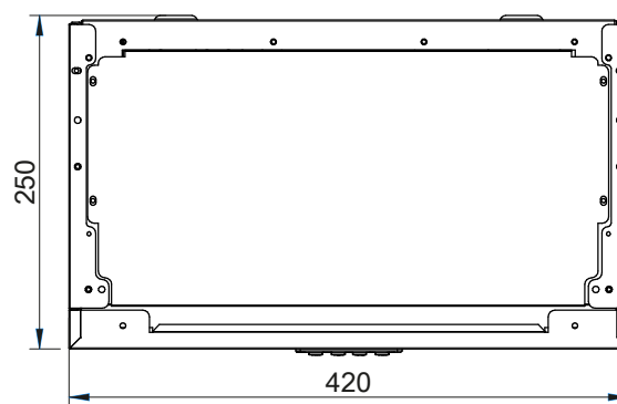
fig. 12 - Vista dall'alto
