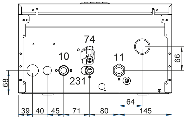
11. ábra - Alulnézet
