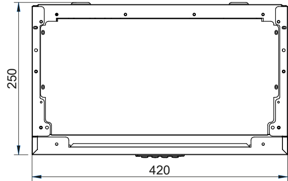
εικ. 12 - Πάνω τμήμα
