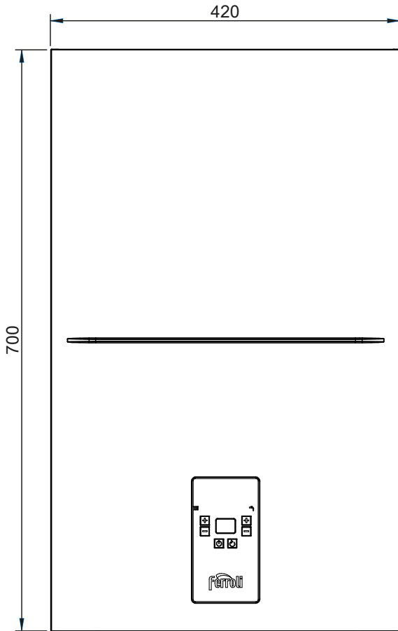
εικ. 9 - Μπροστινό τμήμα
