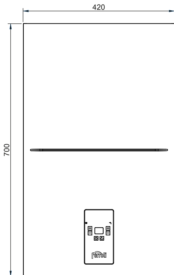
fig. 9 - Vista frontale
